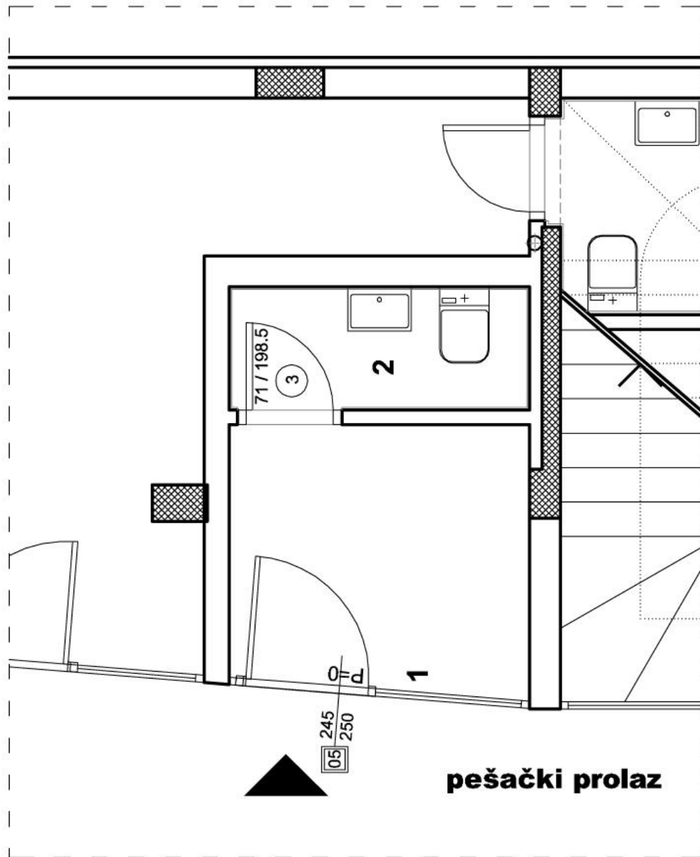
osnova lokala 2 R = 1:100
