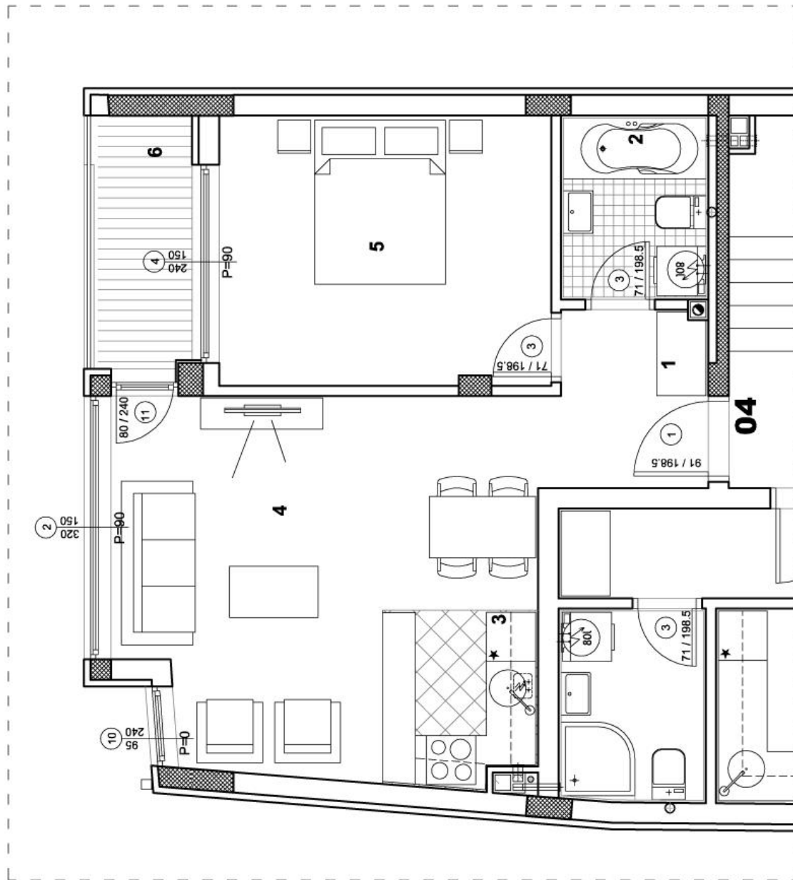
osnova stana R = 1:100
