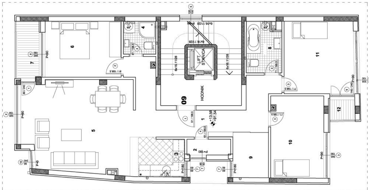
osnova stana R = 1:100
